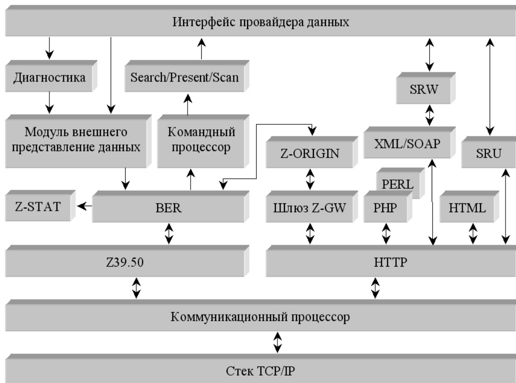
Рис.1. Основные блоки сервера ZooPARK
