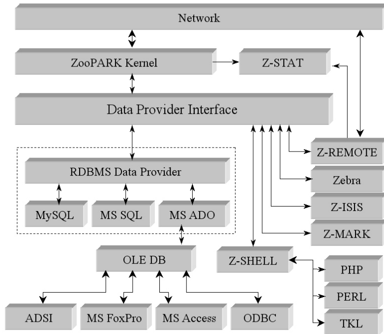
Рис.2 Доступ к данным в сервере ZooPARK
